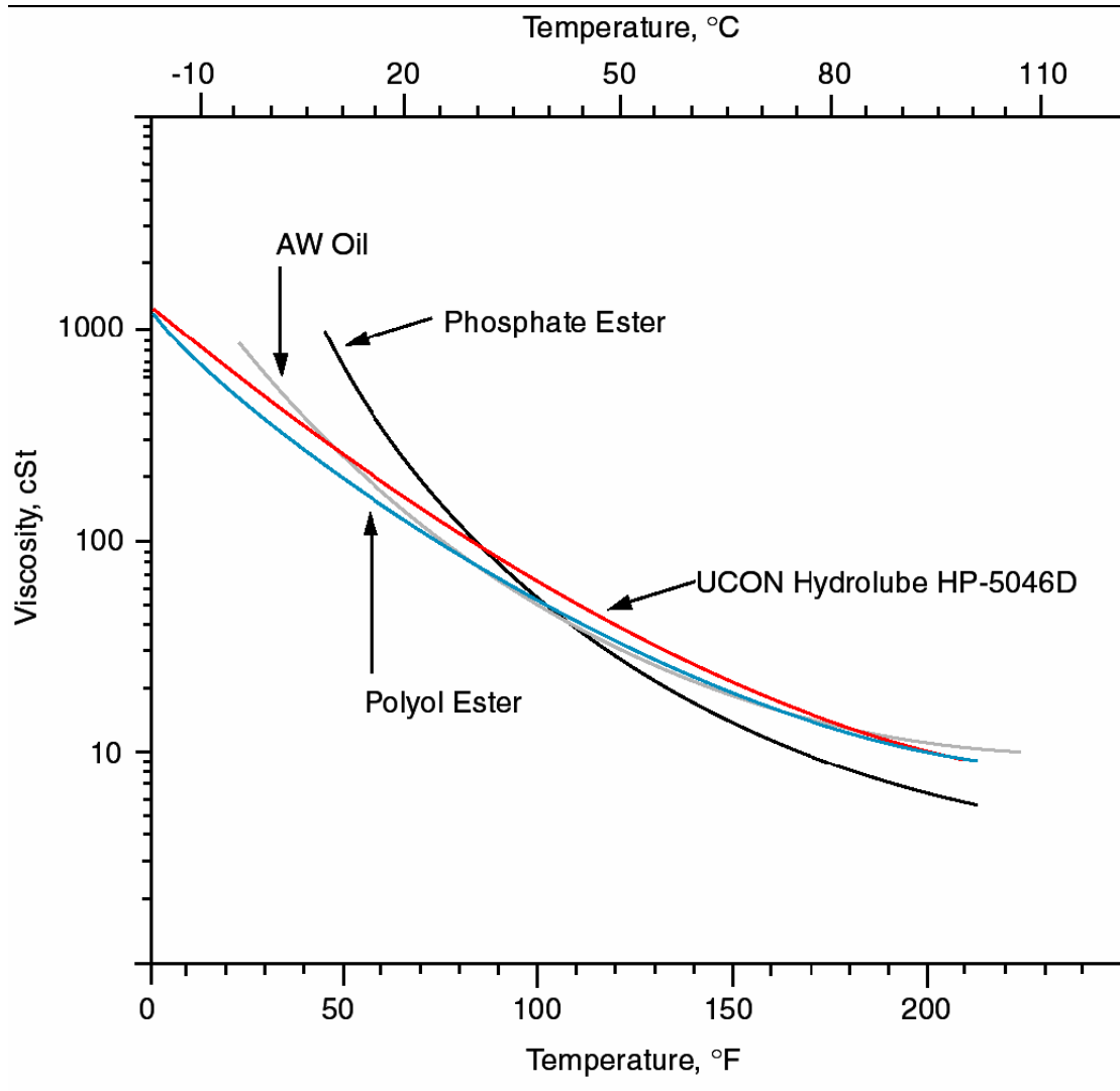
图1. 液压液粘度、温度关系
