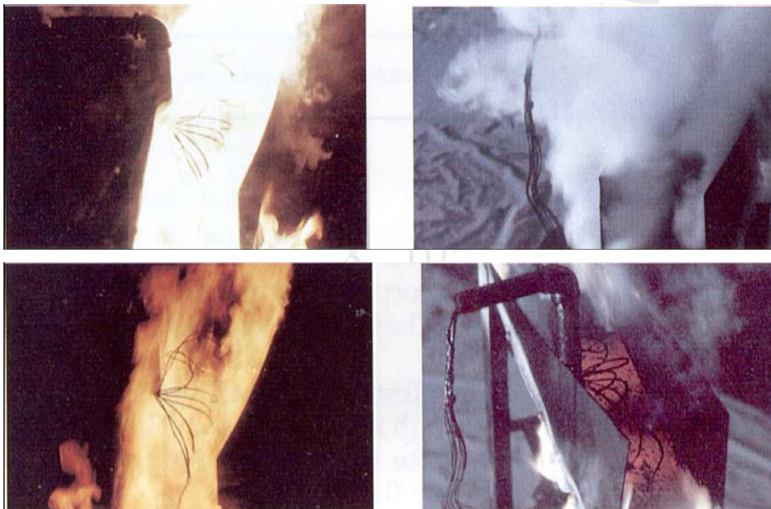
图4 • 各种不同液压液的热管道燃烧测试
